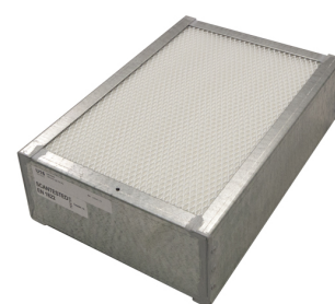
Ulpafilter U16, Abm.: 337 x 230 x 100 mm Artikel-Nr.: 100350005
